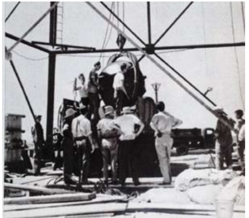
L'ordigno battezzato "Jumbo" (dal nome di un elefantino dei fumetti) viene issato in cima al traliccio. Gli scienziati assisterono all'esplosione dieci chilometri lontano, dentro un bunker di cemento armato
